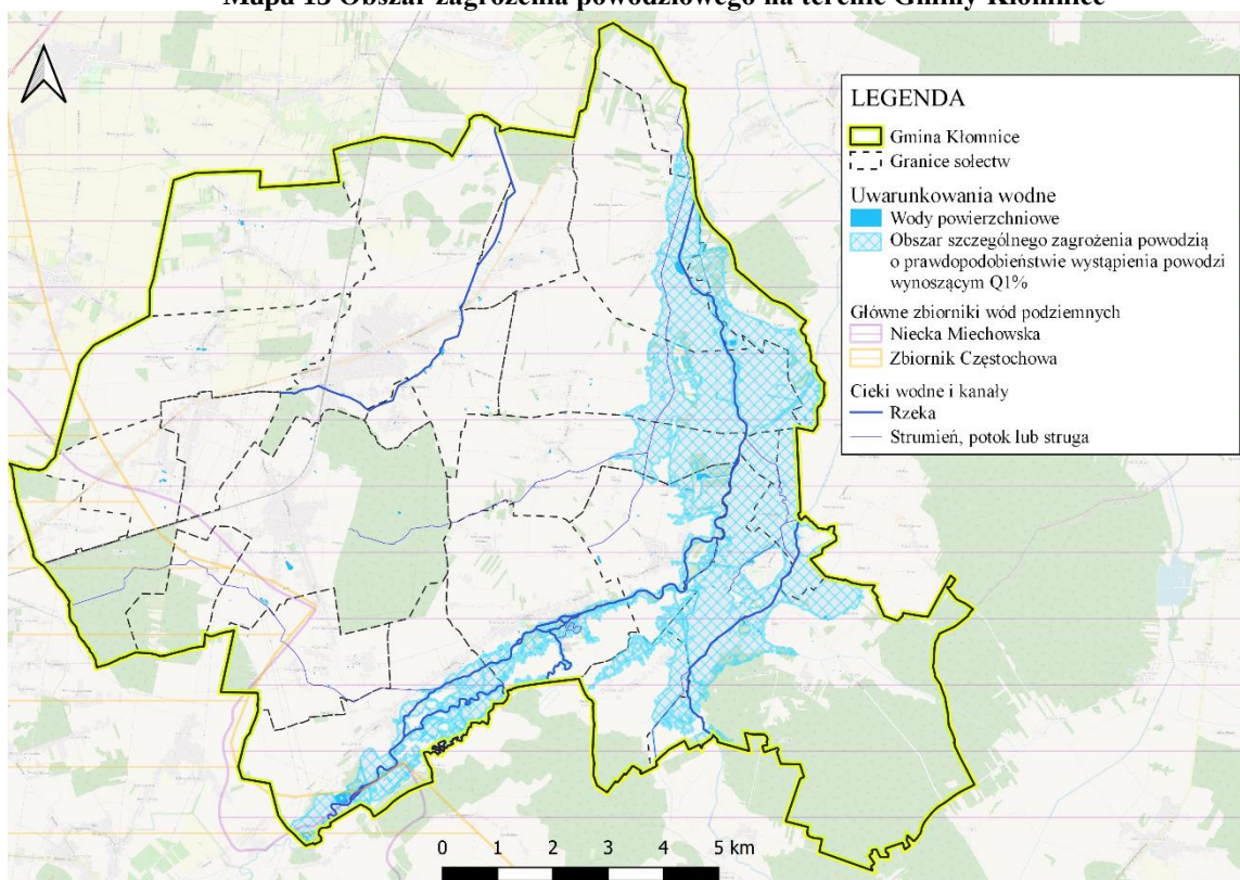
Mapa 13 Obszar zagrożenia powodziowego na terenie Gminy Kłomnice
